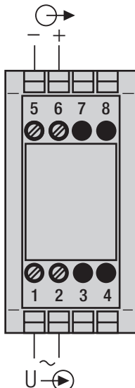
Bild 2. SINEAX U 543, für Wechselspannungs-Messung.
